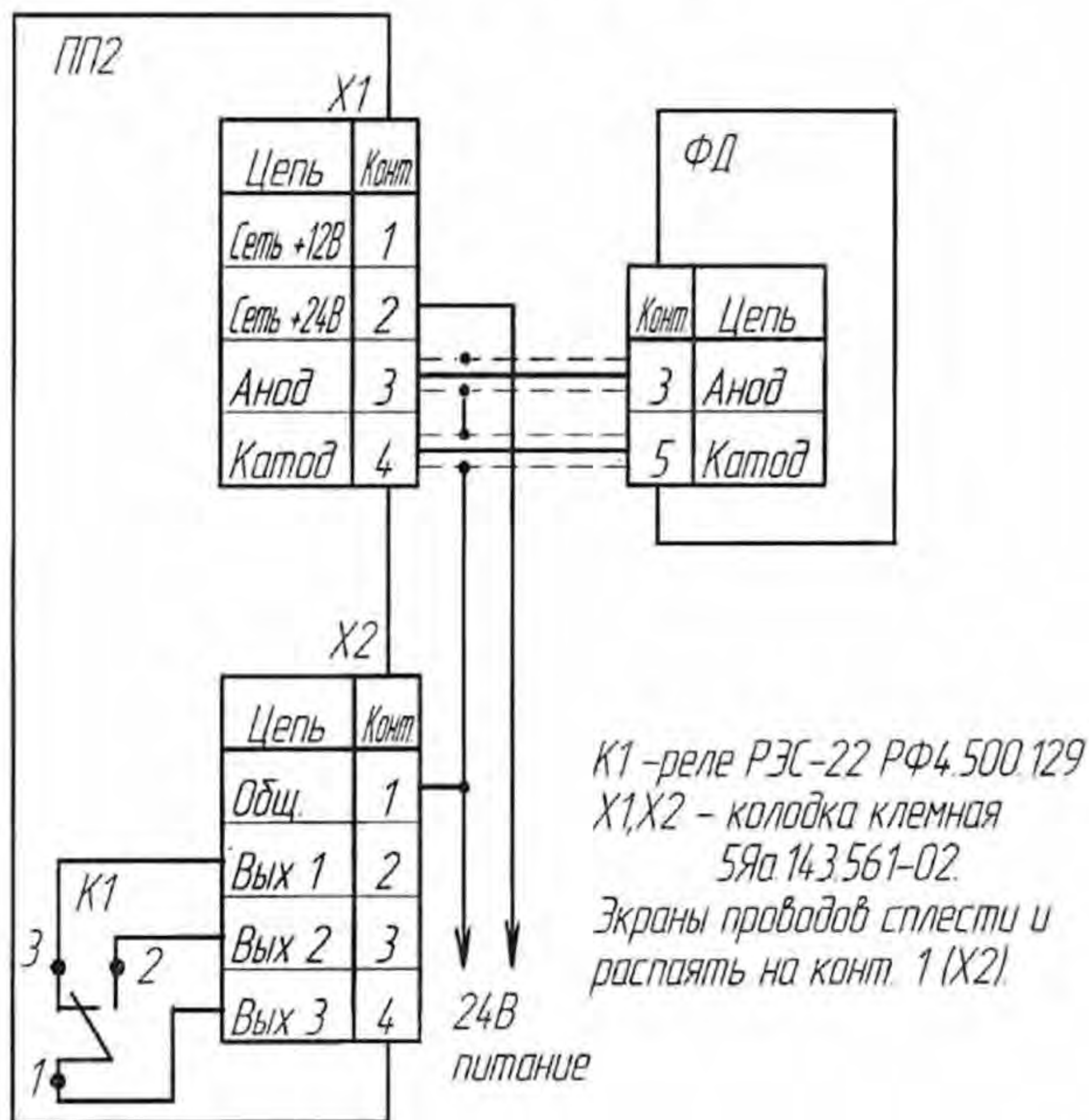
Схема подключения Пламя-M02
