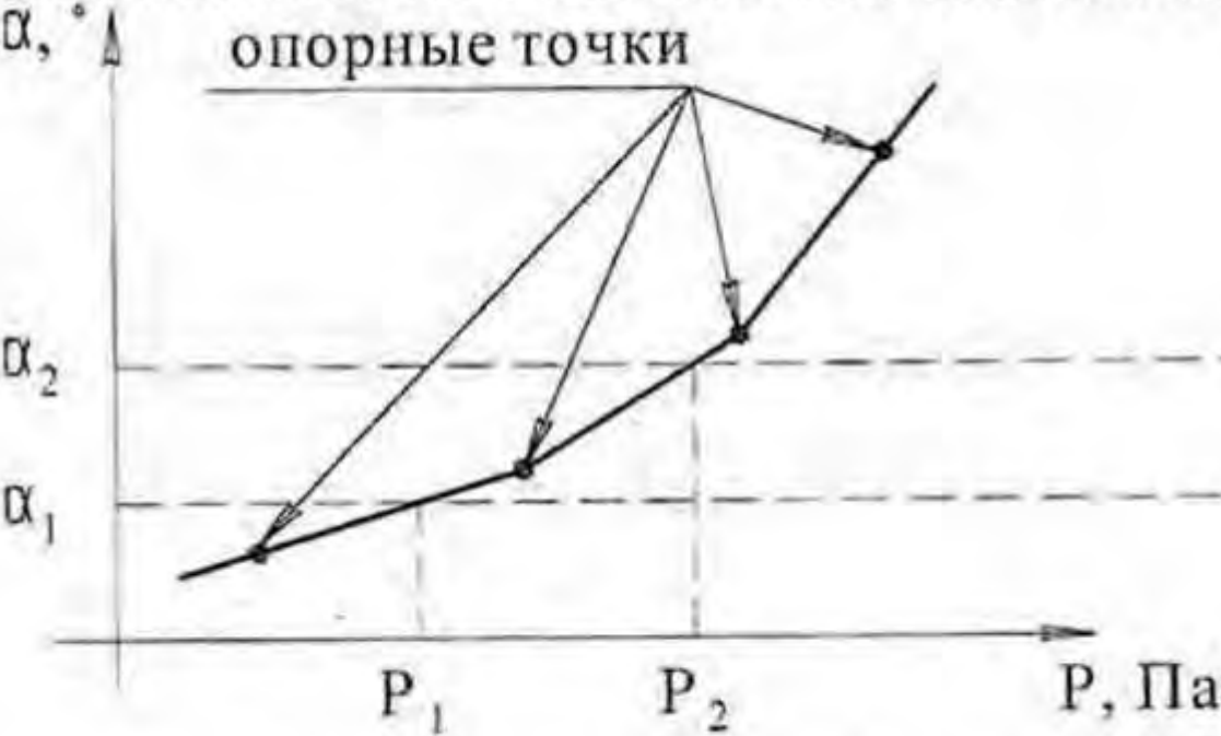
Формирование направляющего напряжения при регулировании
