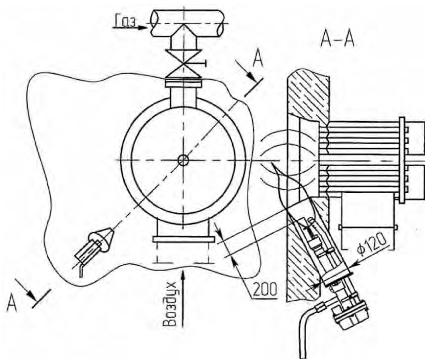
Установка запальника на подовой газовой горелке
