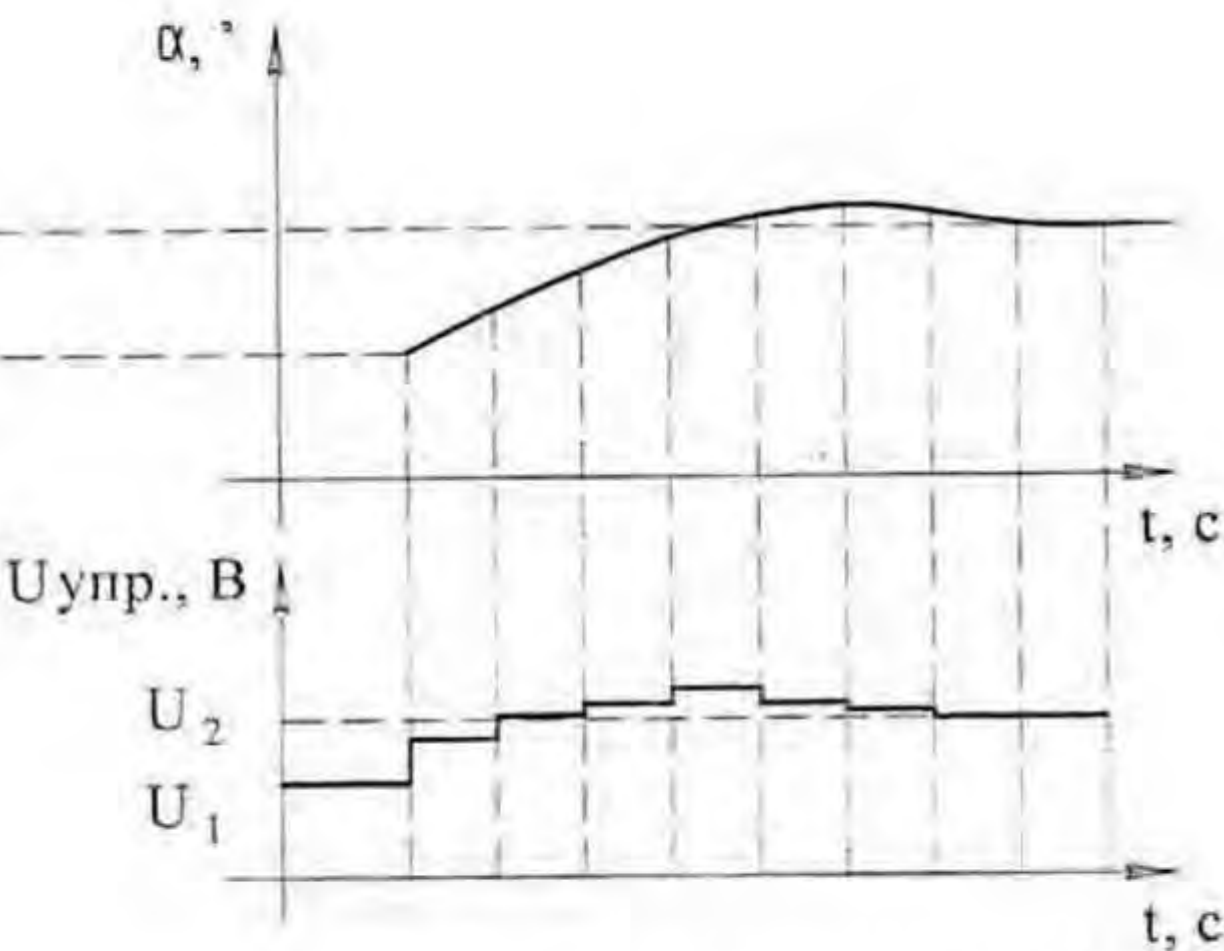
U_{упр.} - напряжение управления МЭО
