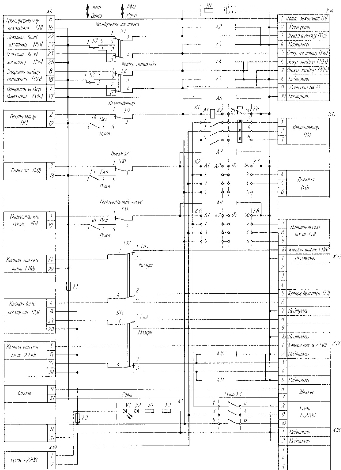
Рис. К. 1 Схема электрическая принципиальная блока БКЭ2
