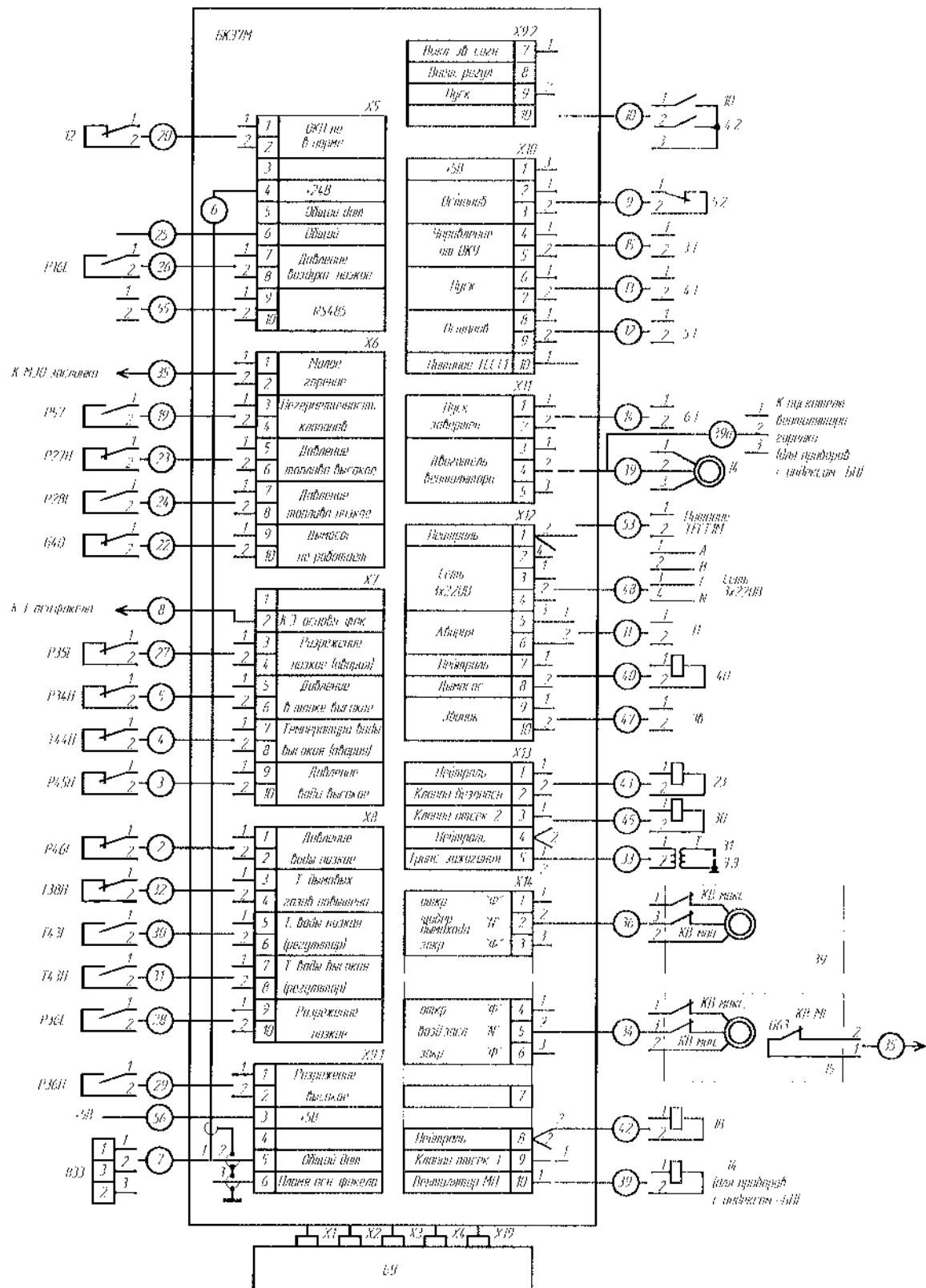
Рис. Н.1 Схема подключения БКЭ7М.
