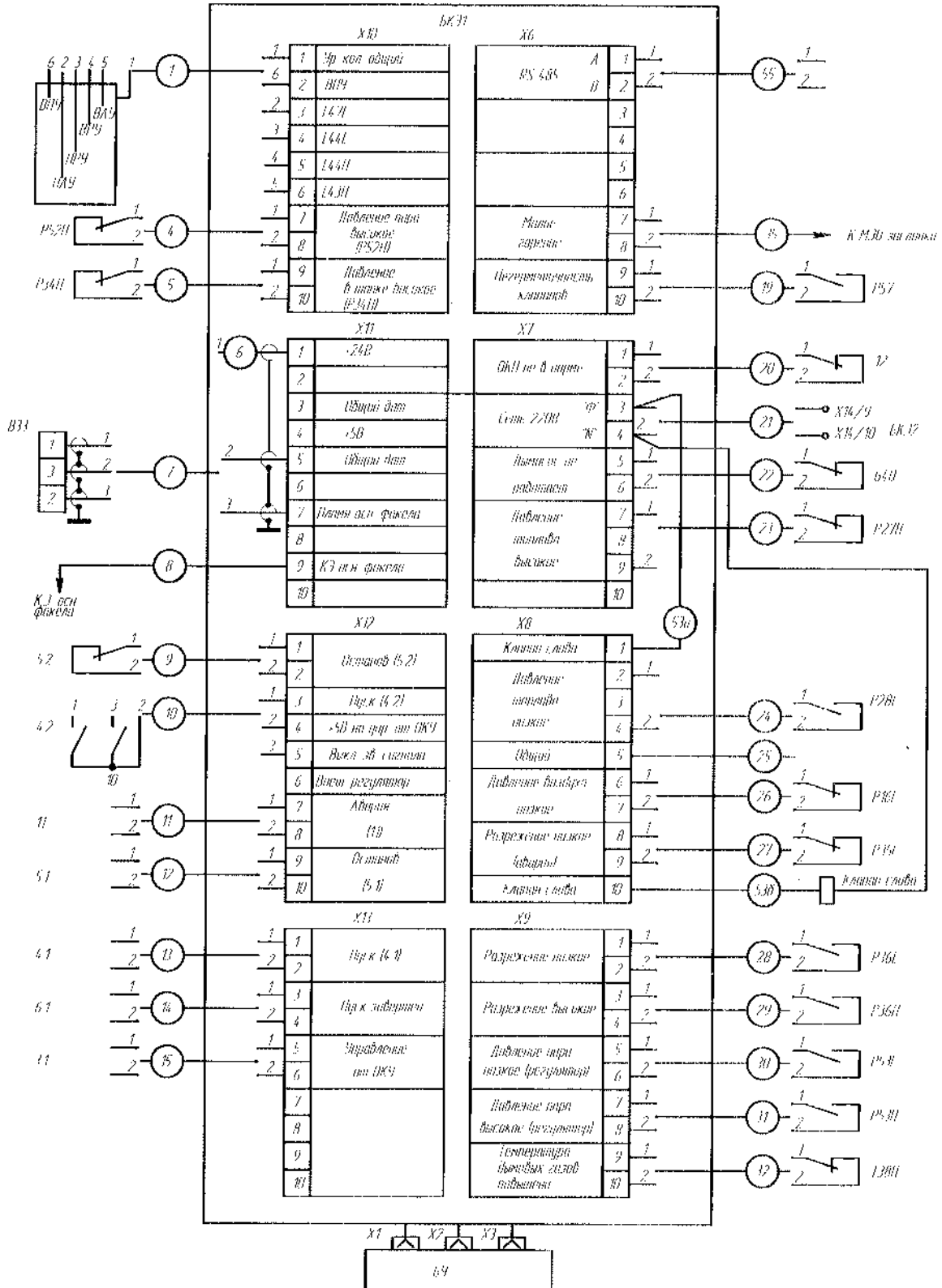
Рис. Н.2 Схема подключения БКЭ1.
