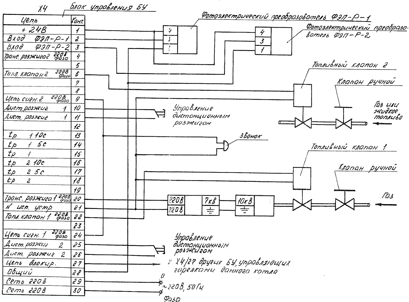
Схема подключения комплекта КРЧК-2-00 при совместной работе загляльника и горелки.
