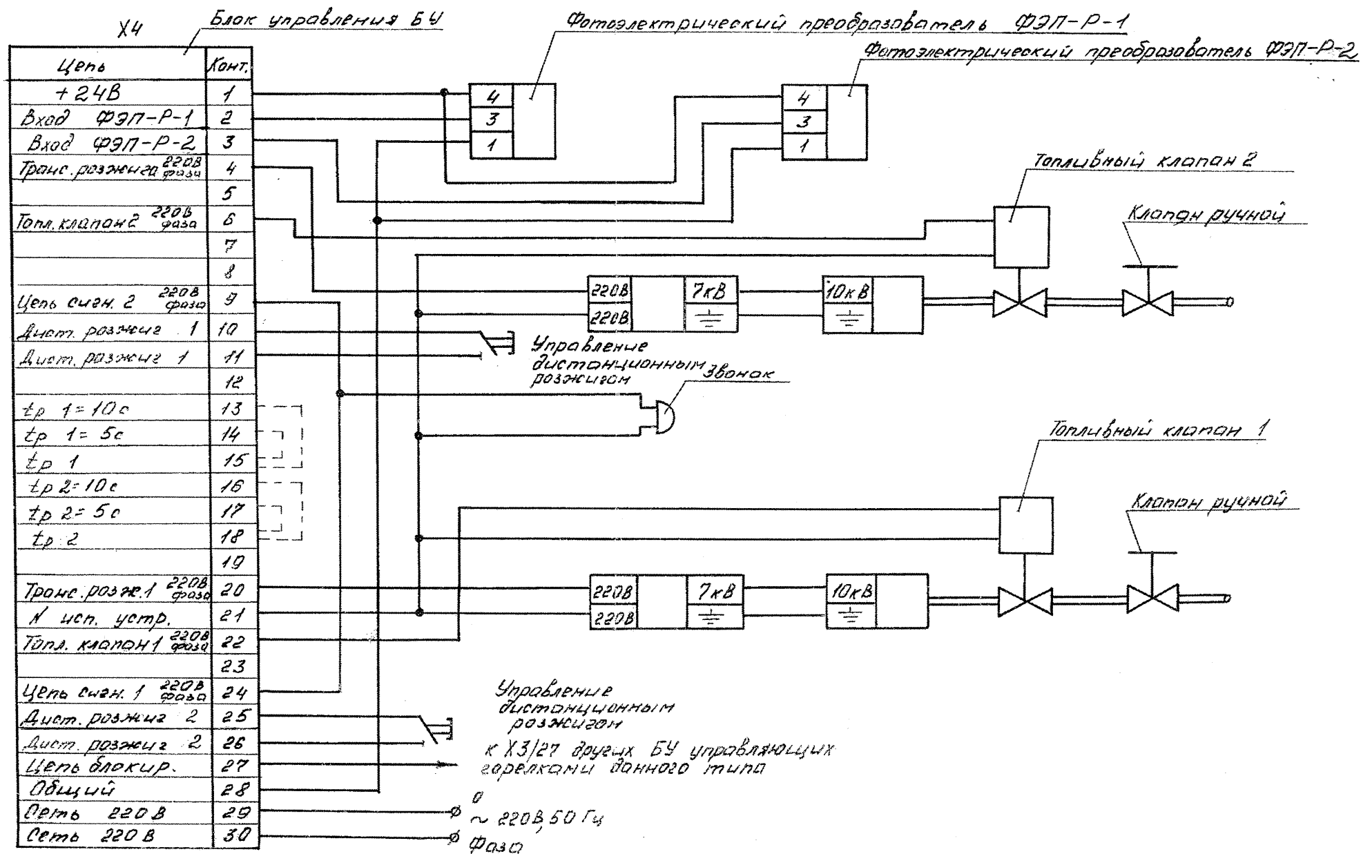
Схема подключения комплекта КРЦК-2-01 при работе с двумя запальниками
